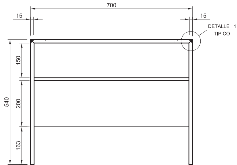
MODULO E - ELEVACION FRONTAL -
