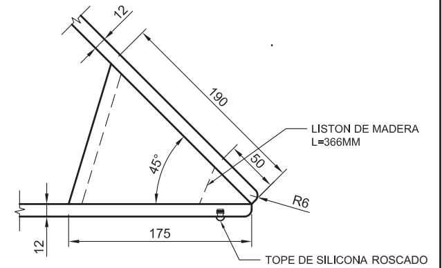
DETALLE 5 Esc: 1/5
