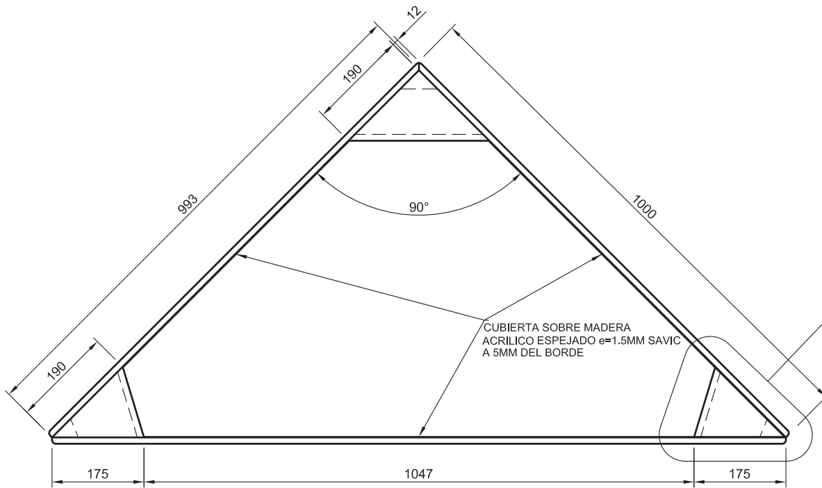
MODULO I - ELEVACION FRONTAL -
