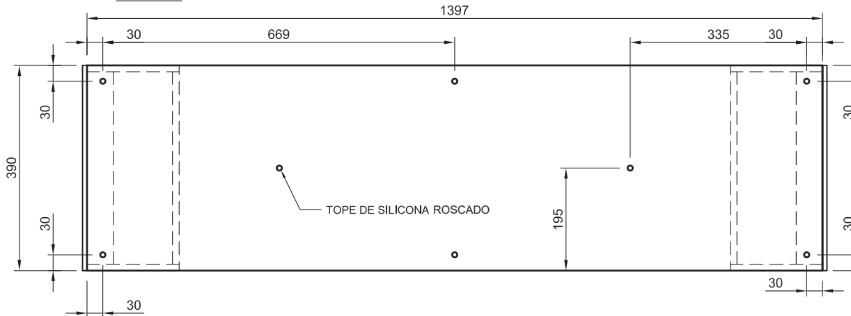
MODULO I - VISTA INFERIOR -
