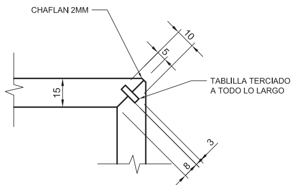
DETALLE 3 Esc: 1/2
