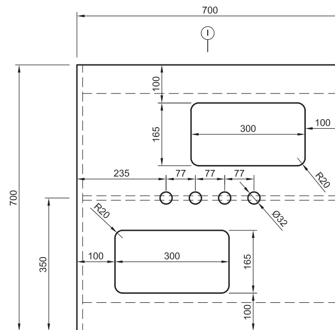
MODULO D - PLANTA -
