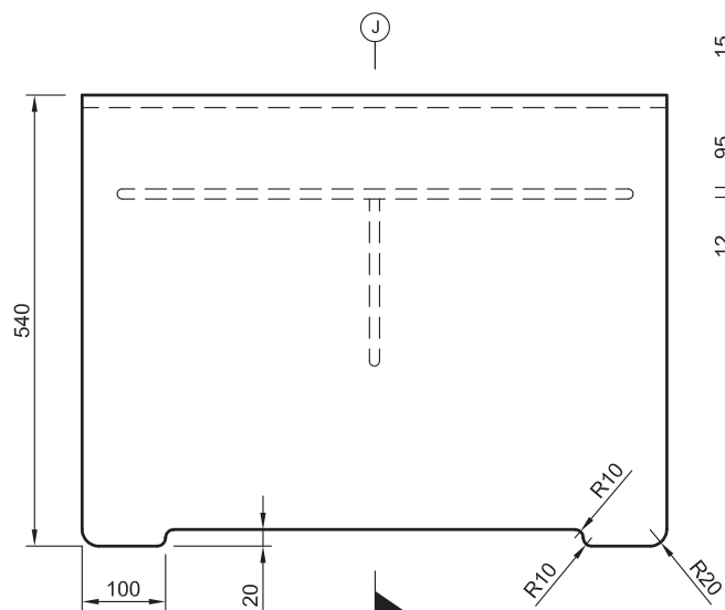
MODULO D - PERFIL -
