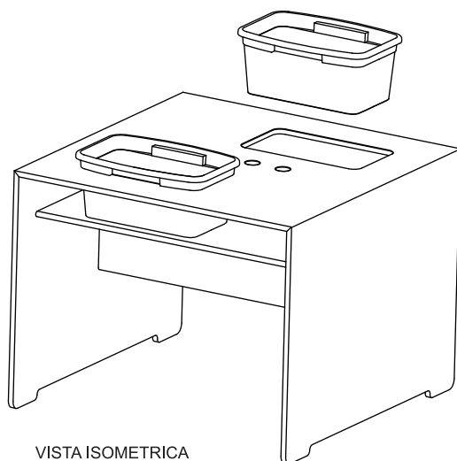
VISTA ISOMETRICA Sin Esc.
