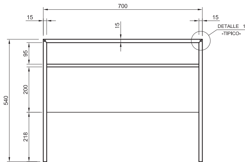
MODULO D - ELEVACION FRONTAL -
