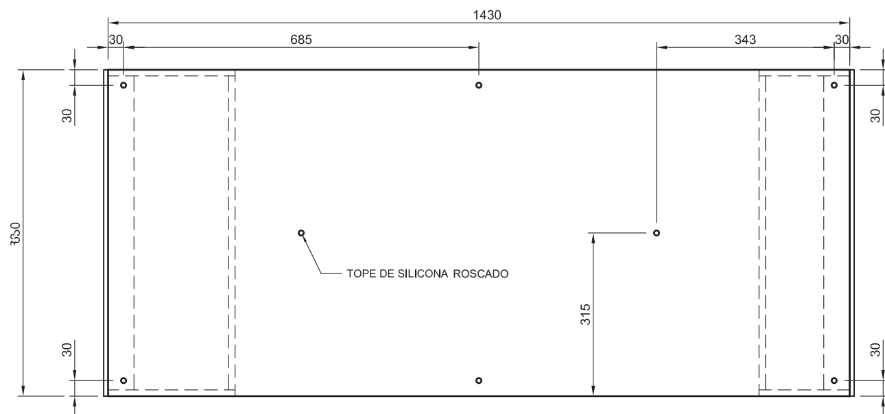
MODULO K - VISTA INFERIOR -
