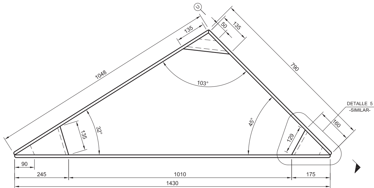
MODULO K - ELEVACION -
